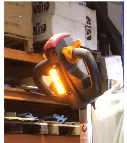
Voyant clignotant N/P : 3601515ass Dimensions: 120 x 40 x 30 mm
